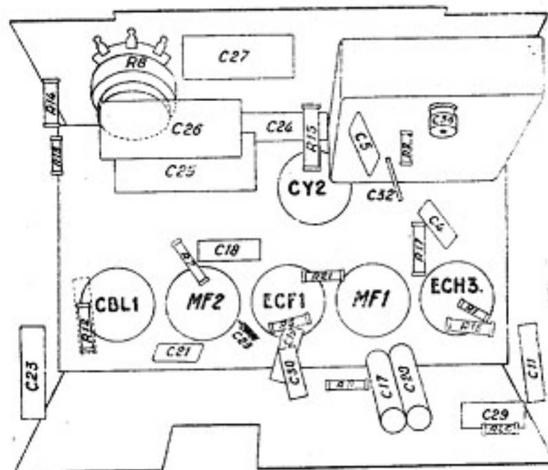
Disposition des pièces, résistances et capacités, à l'intérieur du châssis A43UB.
