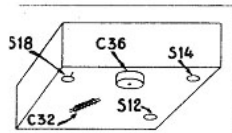
Disposition des condensateurs et des noyaux ajustables sur le bloc de bobinages.
