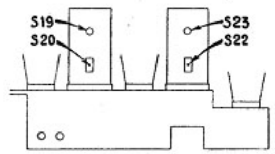
Disposition des noyaux ajustables sur les transformateurs M.F.
